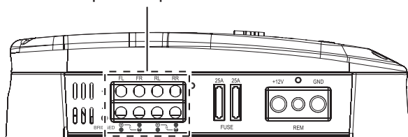
Подключение громкоговорителей
